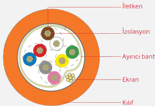
Kablo yapısı
